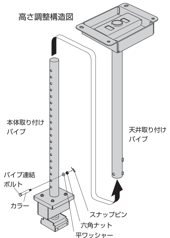
●高さ調整範囲(20段階) (単位 mm)
