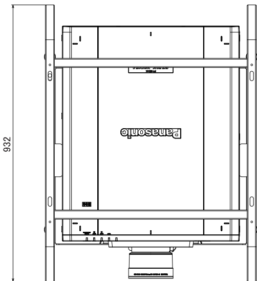
<本金具を組み立て、PT-RQ22K/RZ21K/RS20Kを装着した図>
