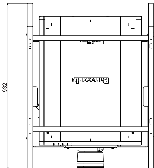
<本金具を組み立て、PT-RQ13K/RZ12K/RS11Kを装着した図>
