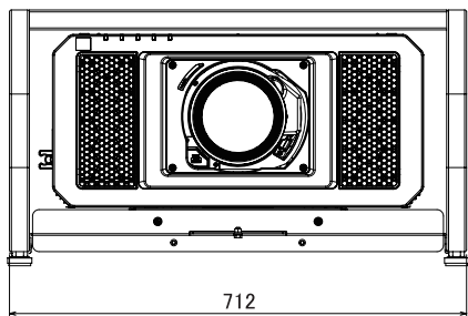
<本金具を組み立て、PT-RQ22K/RZ21K/RS20Kを装着した図>
