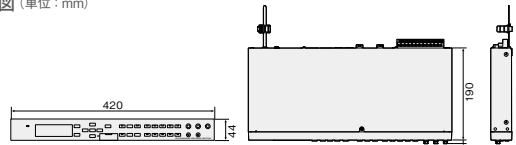
■寸法図 (単位: mm)
