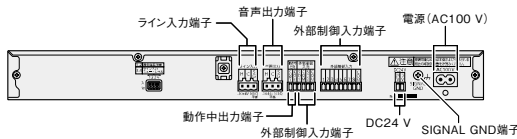
■ 背面パネル
