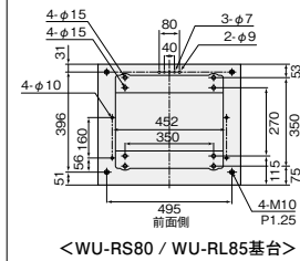
■ 寸法図 (単位: mm)
