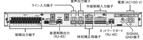
■ 背面パネル
