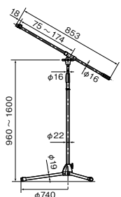
■ 寸法図 (単位: mm)
