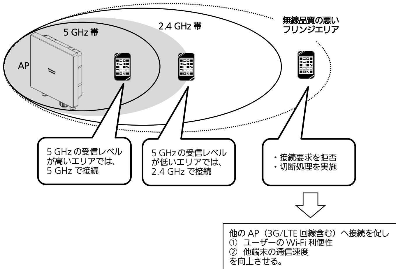
図1.2-5 無線通信品質向上イメージ
