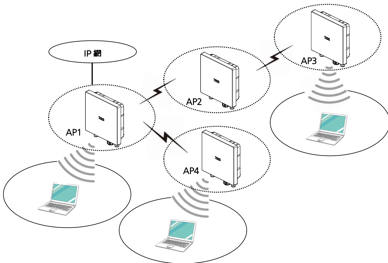
図4.10-1 構成例（無線ブリッジ）
