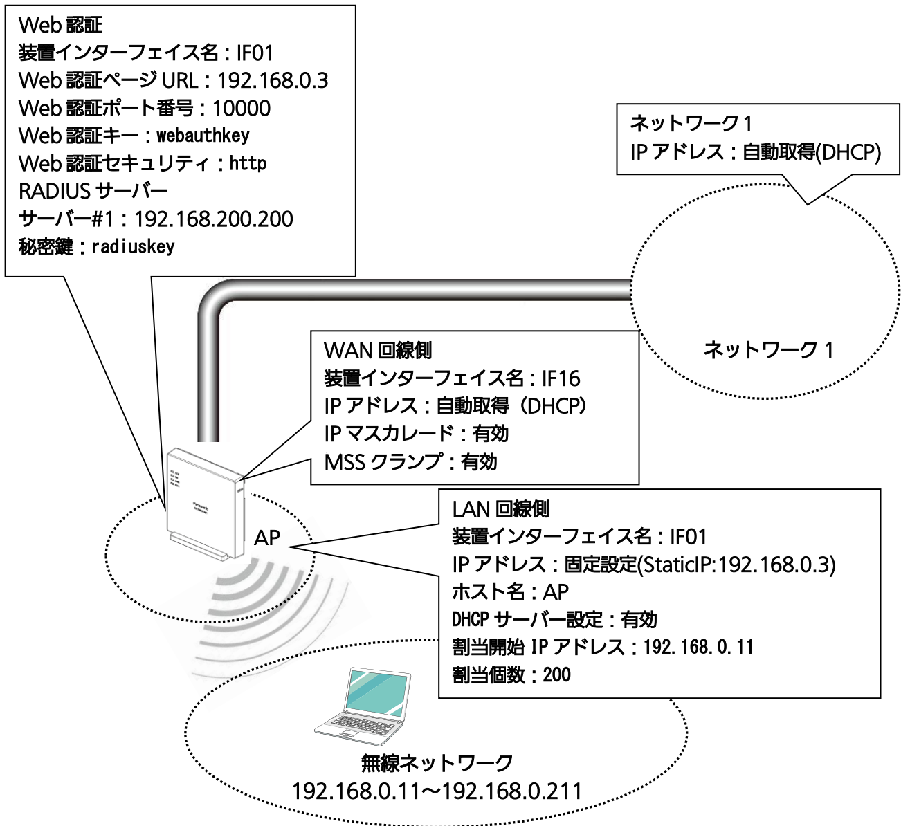
図5.6-1 ネットワーク構成例 (Web 認証)
