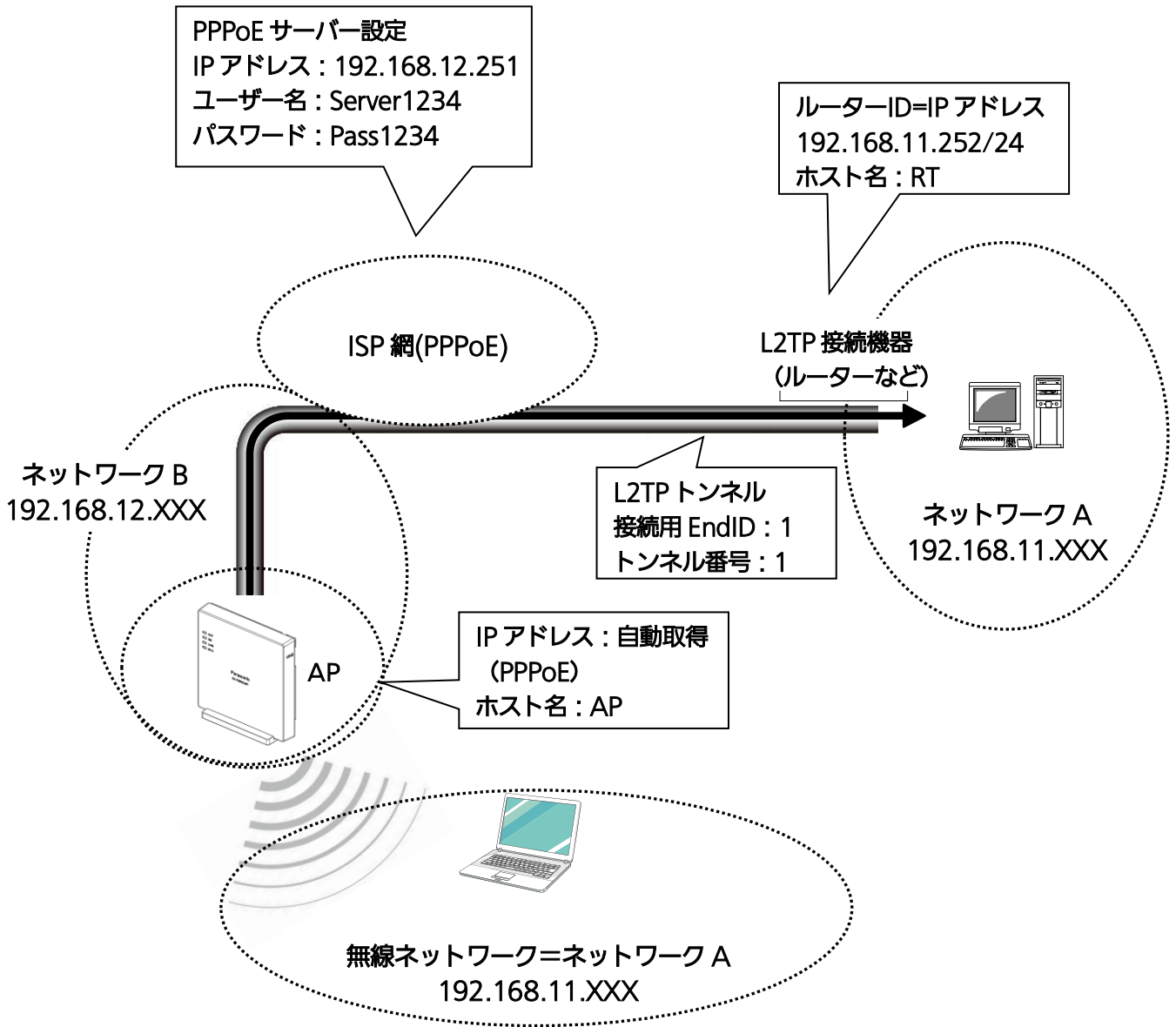
図5.1-1 ネットワーク構成例 (L2TP over PPPoE)
