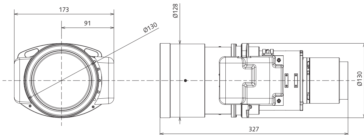
[PT-MZ17KJL/PT-MZ14KJL/PT-MZ11KJL/PT-MZ16KJL/PT-MZ13KJL/PT-MZ10KJL] のプロジェクターに装着した図
