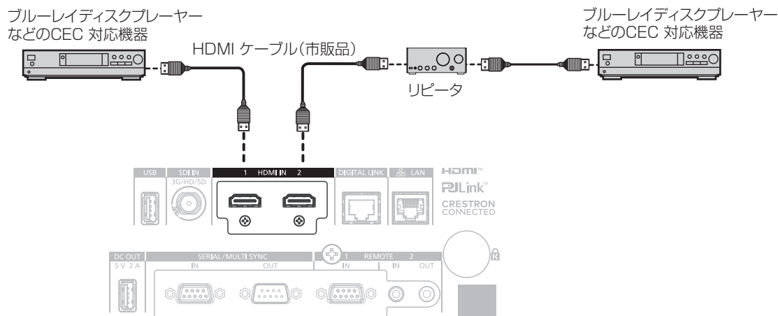
CEC 対応機器との接続（例）
