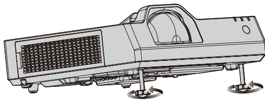
最大調整可能量 各アジャスター脚：30 mm
