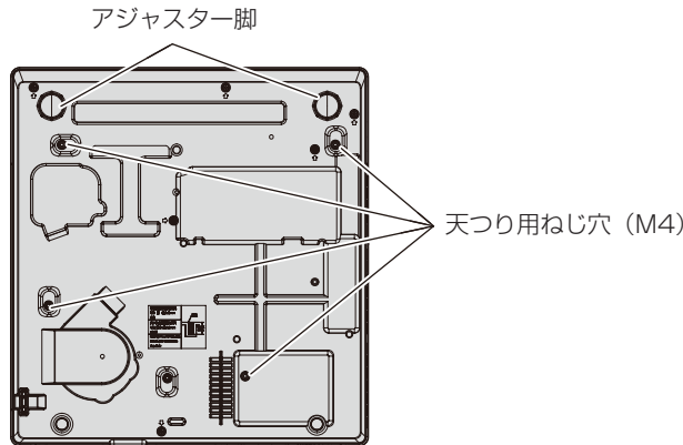
天つり用ねじ穴 (M4) とアジャスター脚の位置
