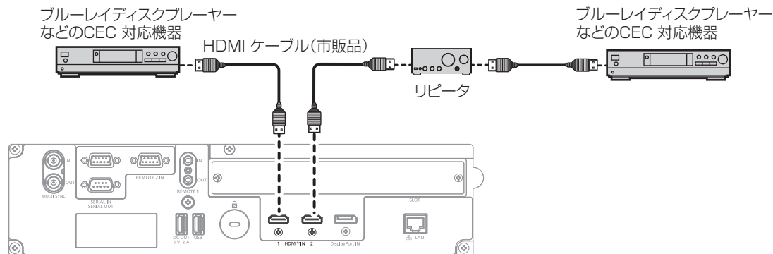
CEC 対応機器との接続（例）
