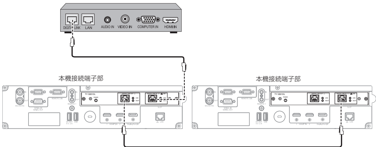
ツイストペアケーブル伝送器の例
